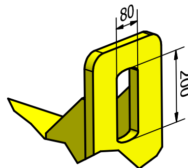
Detalhe A Olhal Superior
