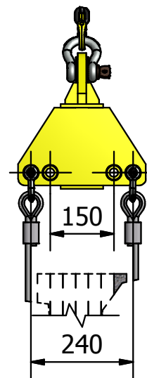
DETALHE A REGULAÇÃO DA POSIÇÃO
